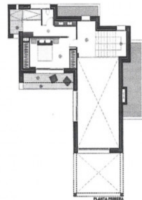
PLANTA PRIMERA
