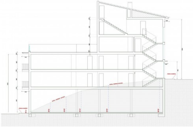
SECCIÓN A-A'
